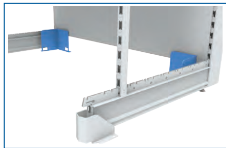
2 Odbojnik palety Pallet guard • Butée • Abweiser • Отбойник
