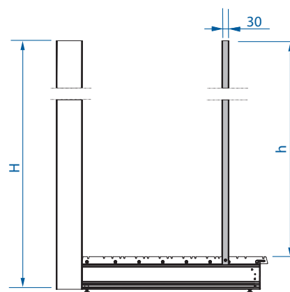
3 FRONT 30 × 30 Stup • Add-on upright • Montant • Säule • Профиль
