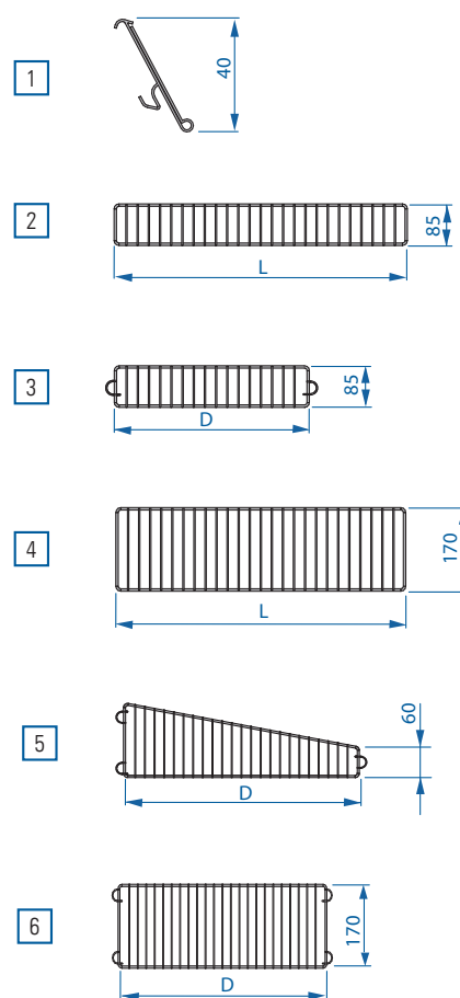
3 WIRE H-85 • Przegroda • Divider Séparateur • Trenngitter • Перегородка
