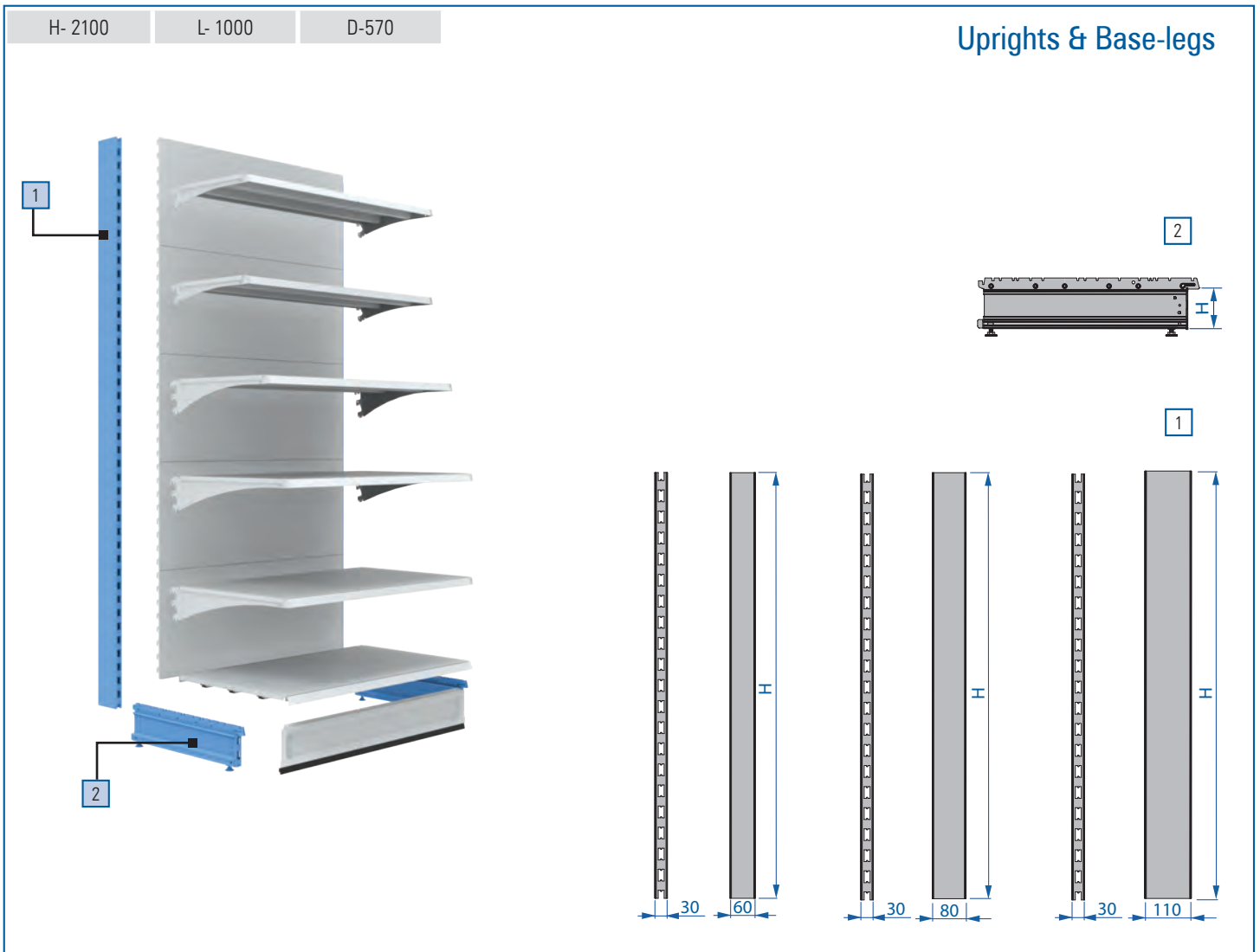
1 60 × 30 Slup • Upright • Montant • Säule • Профиль
