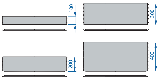
2 Osłona dolna • Plinth Plinthe • Sockelblende • Плинтус
