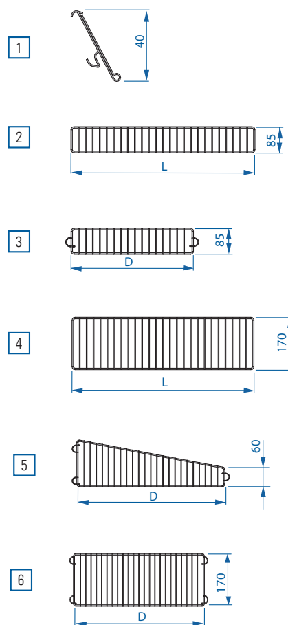
3 WIRE H-85 • Przegroda • Divider Séparateur • Trenngitter • Separatierooster
