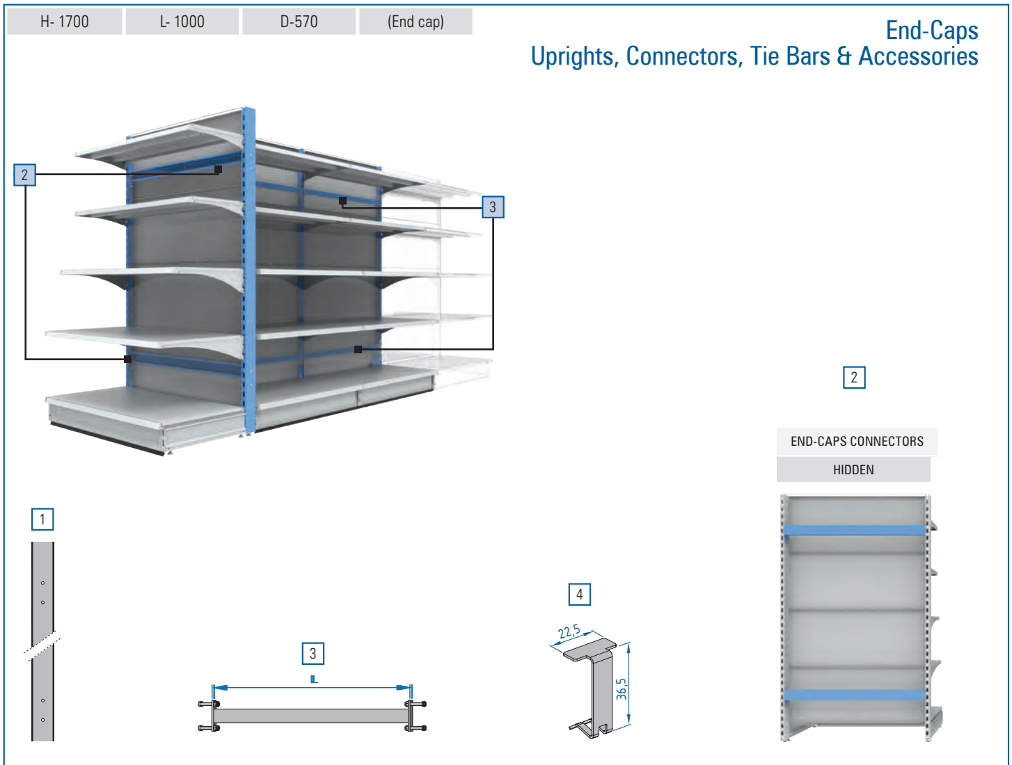
1 60 x 30 DRILLED Slup • Add-on upright • Montant • Säule • Stijl met boorgaten
