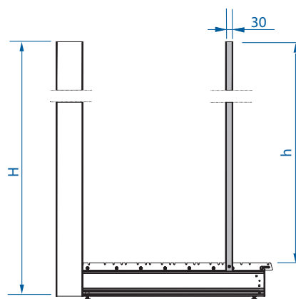
3 FRONT 30 × 30 Stup • Add-on upright • Montant • Säule • Voorzetstijl
