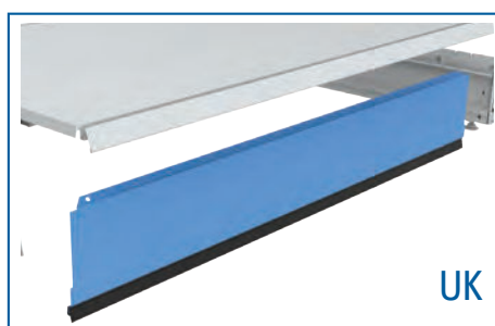
5 UK • Oslona dolna • Plinth • Plinthe Sockelblende • Plint glad
